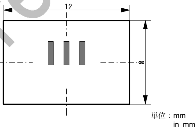
第2図 たわみ試験用プリント基板 Figure 2. PCB for Bending Strength Test
